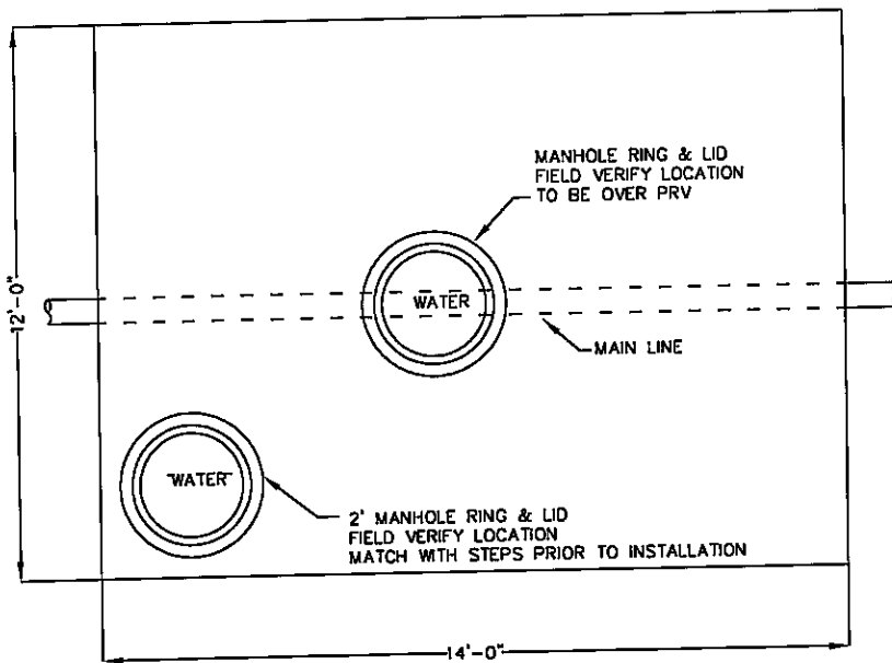
TOP VIEW LID
