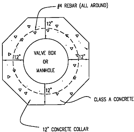
PLAN OPTIONAL
